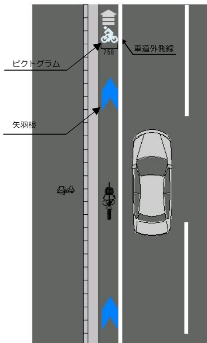
図 4-10 路肩・停車帯内の整備
