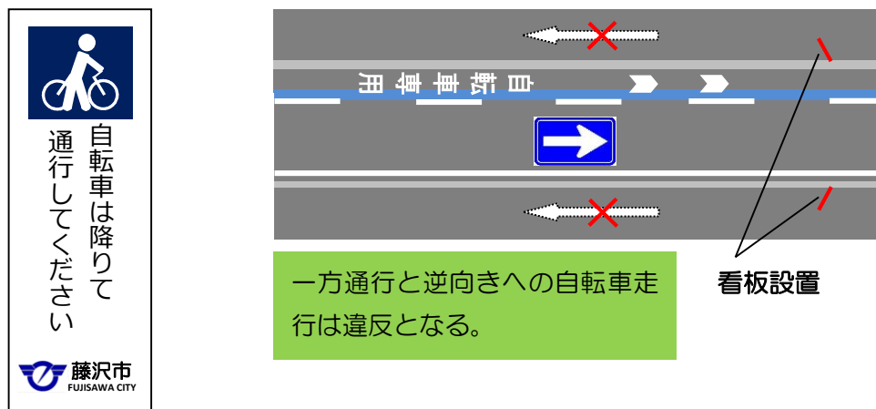
図 4-5 一方通行道路への自転車専用通行帯設置
