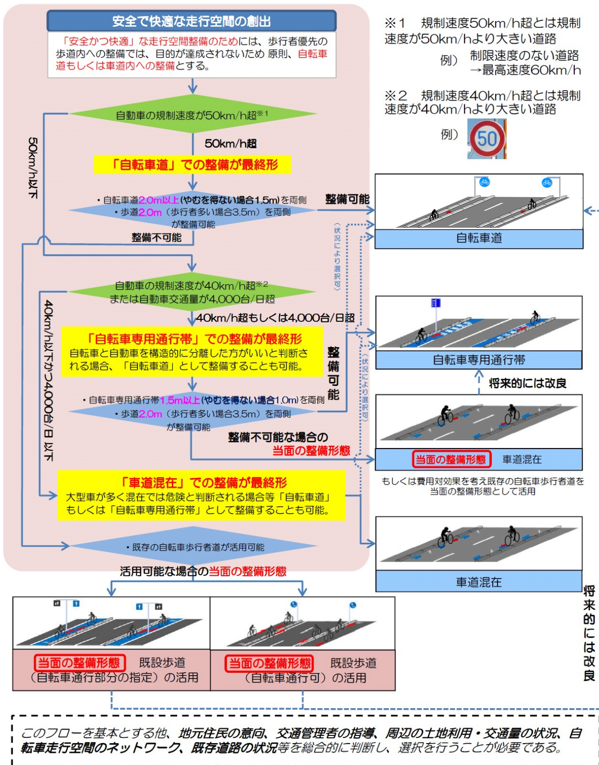
図 4-18 整備形態選択フロー
