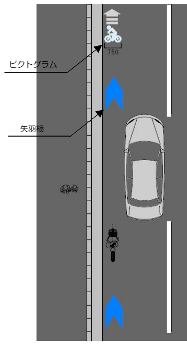
図 4-11 車線内の整備
