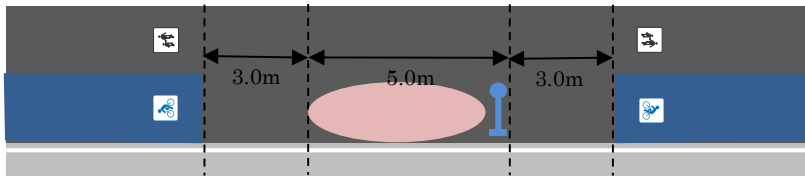
図 5-14 自転車の走行位置の法定外の明示を行わない場所（バス停の手前②）
