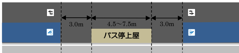
図 5-13 自転車の走行位置の法定外の明示を行わない場所（バス停の手前①）
