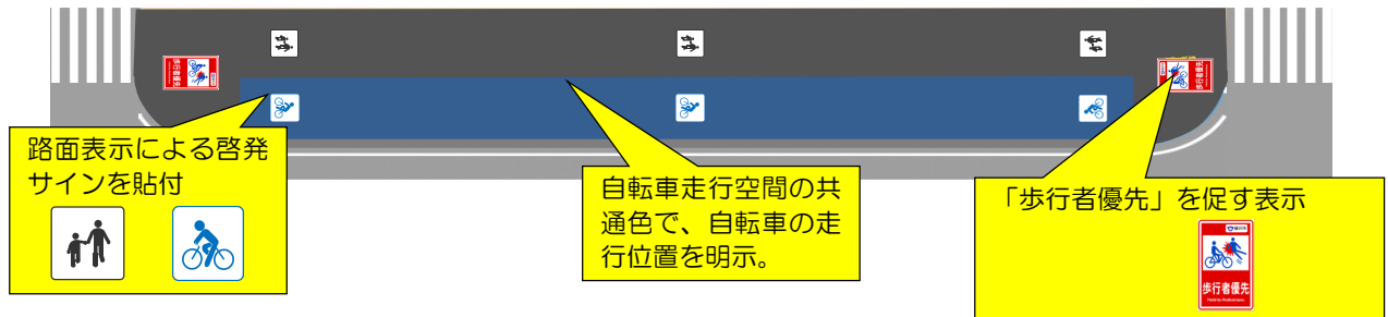
図 4-15 普通自転車歩道通行可の歩道での自転車通行位置の明示
