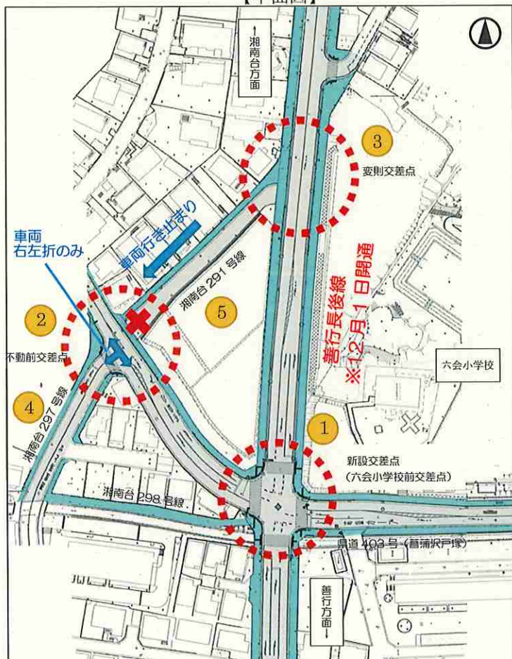
【平面図】
